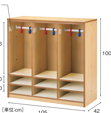
カスタム おしたく収納 6 人用 下段棚板ロッカー
